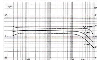
Endstufe
