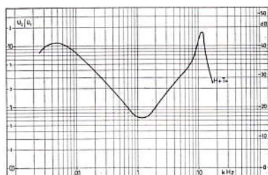
Kanal I/Ia
