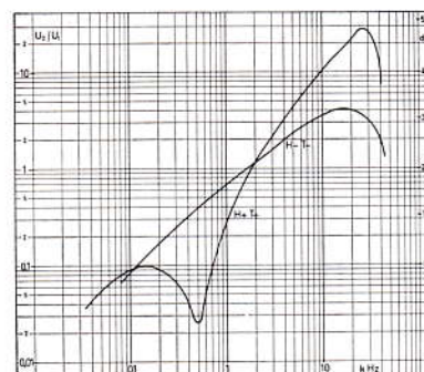
Frequenzgänge:
