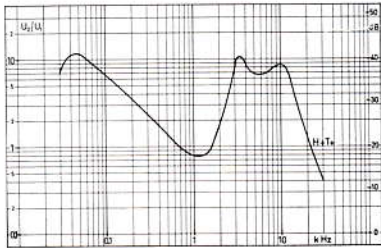
Frequenzgänge:
